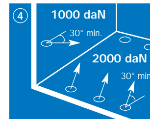
Zurrpunktschild nach DIN EN 12640 (Mindestgröße 200/150 mm)
