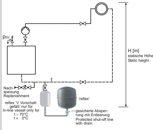
Beispiel Heizungsanlage Example heating system
