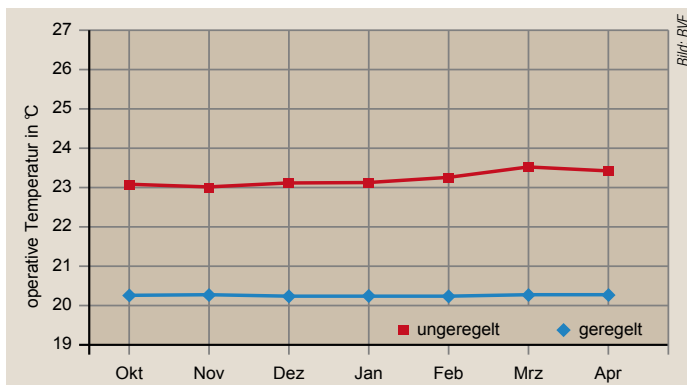
Bild 7 Monatsmittelwerte der operativen Raumtemperatur der Zonen 1, 2, 5, 6, 8, 9, 11 (Geregelte / Ungeregelte Variante H_{vent} = 1,0 ; durchgehender Betrieb).
